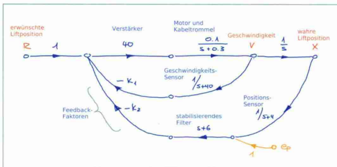
Bild 2: Kommentiertes Signalflussdiagramm eines Feinpositionierungssystems für Lifte
