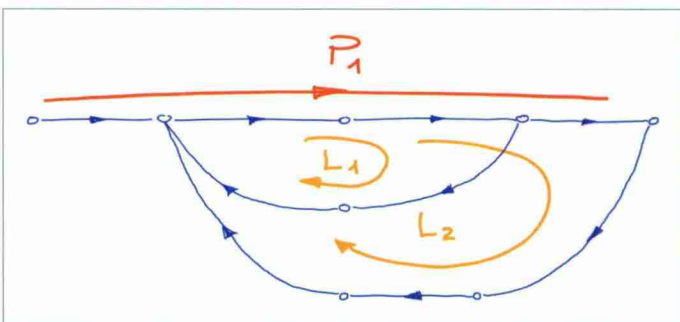
Bild 3: Vorwärtspfad und Kreise im SFD von Bild 2
