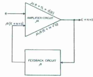
Bild 1: Blacks elektronischer Verstärker aus seinem Paper von 1934 und das zugehörige Signalflussdiagramm (SFD)
