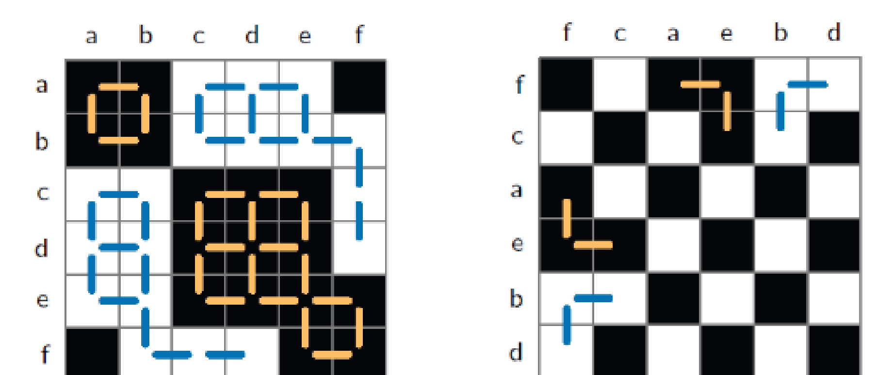
Abb. 5: Adjazenzmatrizen des selben Graphen, mit unterschiedlichen Morans I-Werten (van Beusekom et al. 2022)
