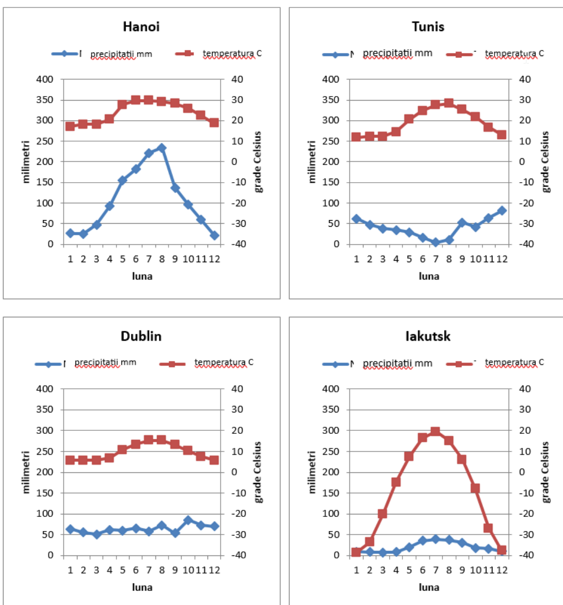
Figura 1. Diagramele climatice sunt alcătuite dintr-o diagramă a precipitațiilor și una a temperaturii. Precipitațiile sunt indicate în stânga, în milimetri, iar temperatura în dreapta, în grade Celsius. Diagramele arată valorile medii ale precipitațiilor și temperaturii din ianuarie până în decembrie.
